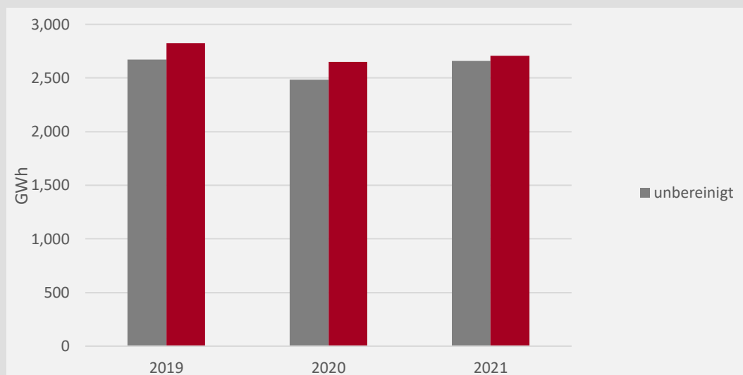
Abbildung 14: Vergleich Endenergieverbrauch witterungsberreinig und unbereinigt für die Jahre 2019 bis 2021
