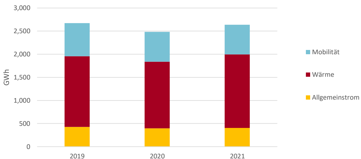
Abbildung 12: Entwicklung des Endenergieverbrauchs nach Anwendungen im Unstrut-Hainich-Kreis
